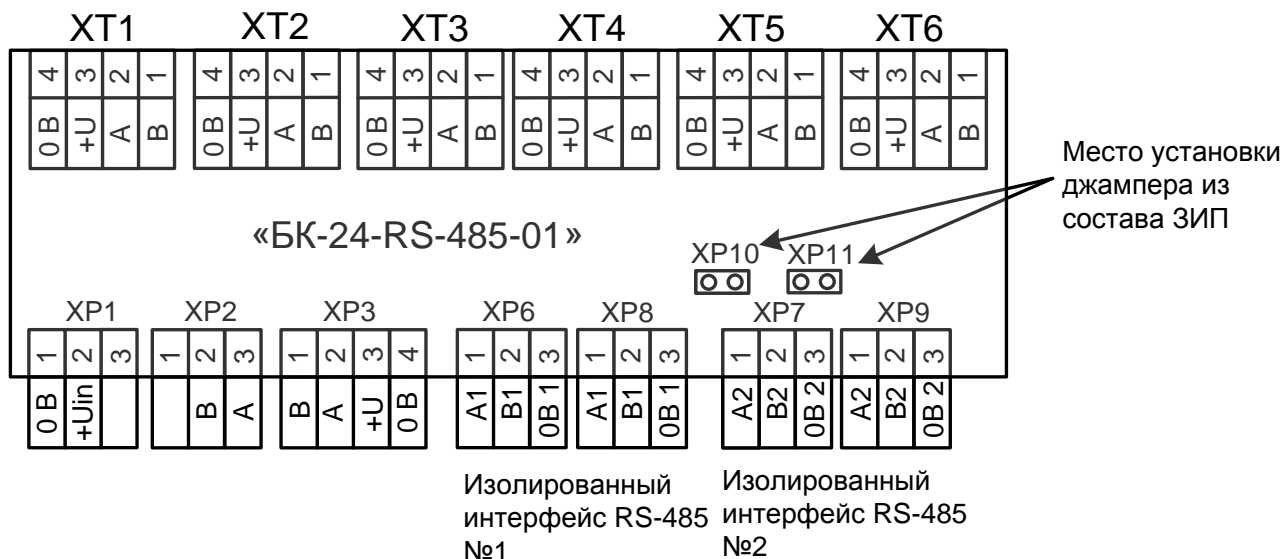
БК-24-RS-485-01 с открытой крышкой
